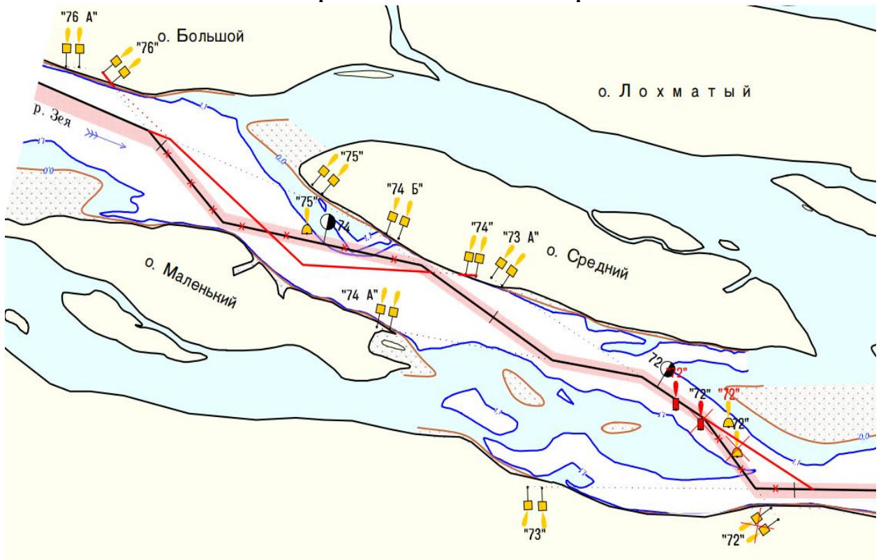
Схема расстановки СНО 76-71 км р. Зейя
